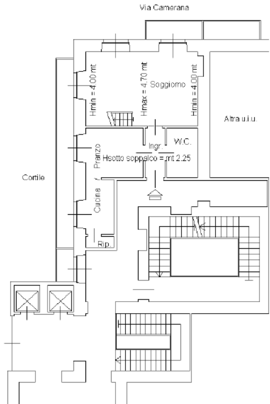
PIANTA PIANO SECONDO (3 f.t.)
